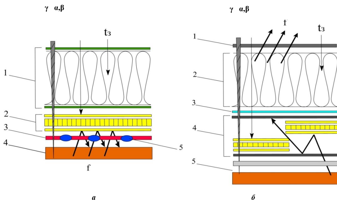
Рис. 2. Схема різновидів пакетів матеріалів в спеціальному одязі для захисту від іонізуючого випромінювання
