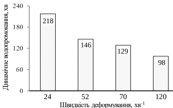
Рисунок 3.4 – Залежність динамічного водопоглинання гідрофобізованої шкіри від швидкості деформування
