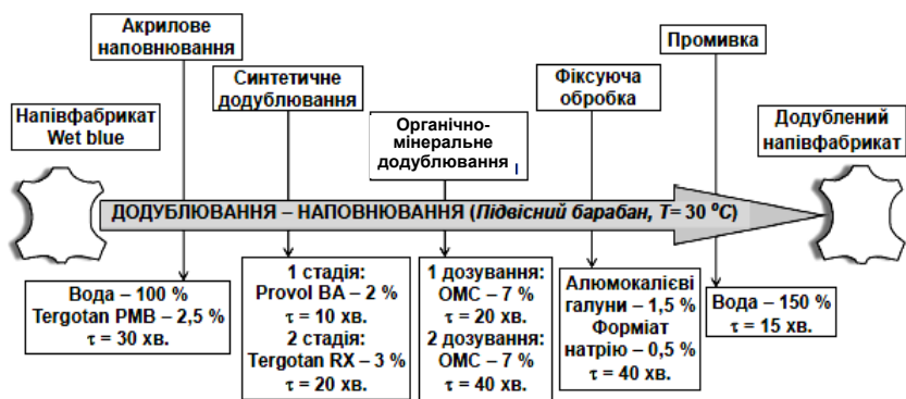
Рисунок 1.5 – Технологічна схема додублювання-наповнювання шкіряного напівфабрикату ОМС
