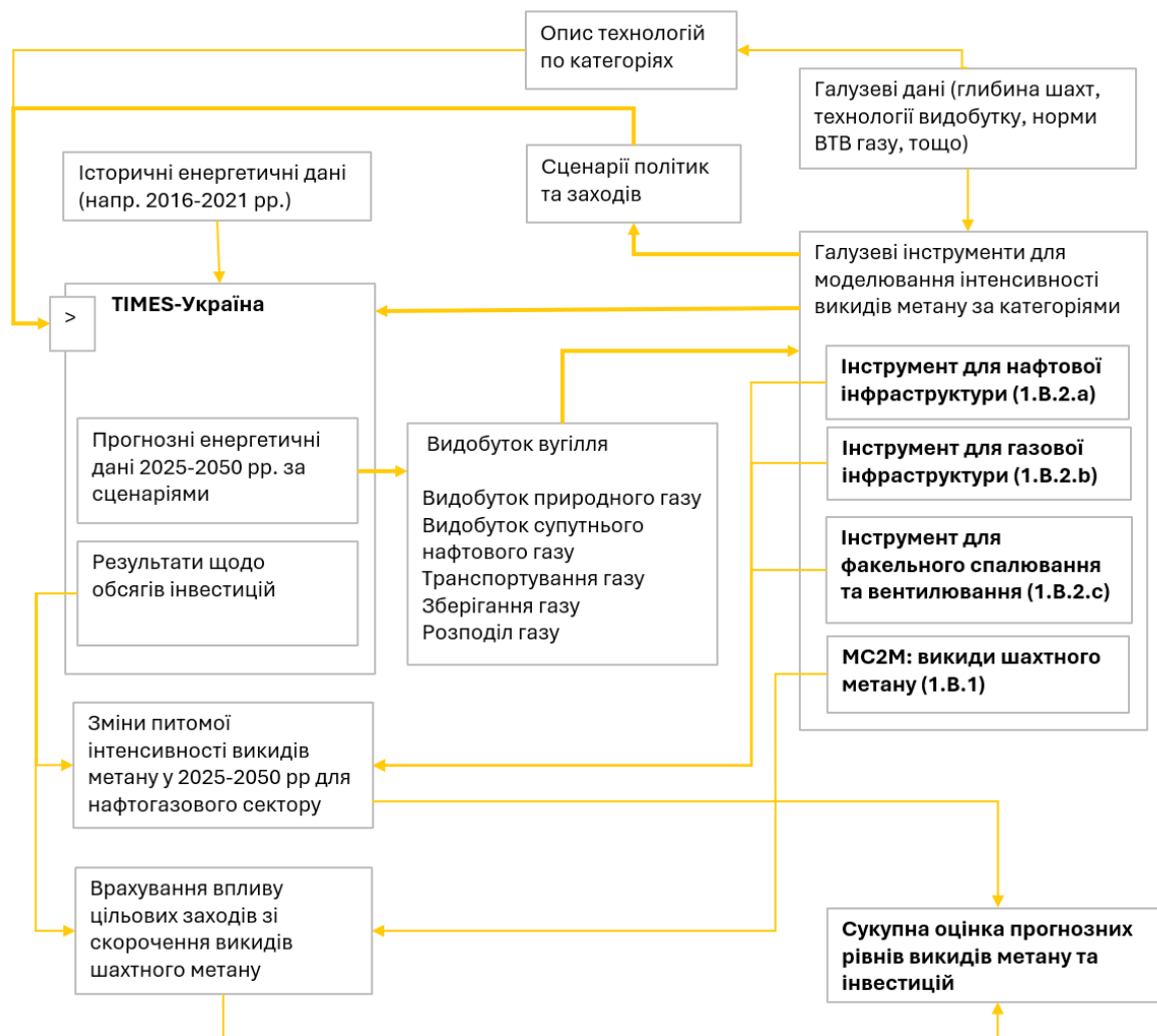
Рис. 1: Схема комплексного модельного інструментарію для сценарної оцінки прогнозних викидів метану та інвестицій.
